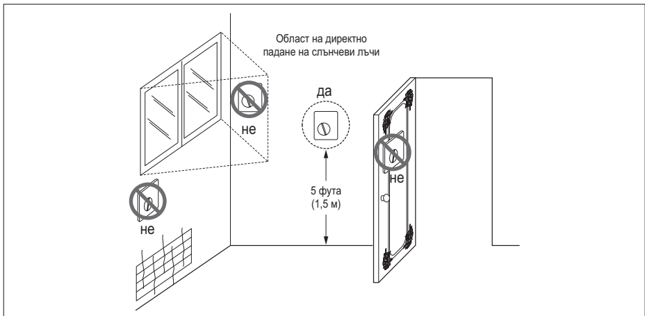
Термостат
