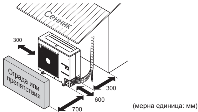
Минимално пространство за обслужване
