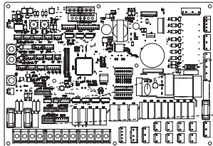
PCB на вътрешно тяло (За Сплит Вътрешно тяло Серия 5, За Хидросплит)
