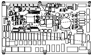
PCB на вътрешно тяло (За Сплит R32 Вътрешно тяло 4 Серия, За Сплит R410A Вътрешно тяло 3 Серия)
