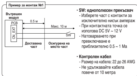
PCB на вътрешно тяло (За Сплит Вътрешно тяло Серия 5, За Хидросплит)
